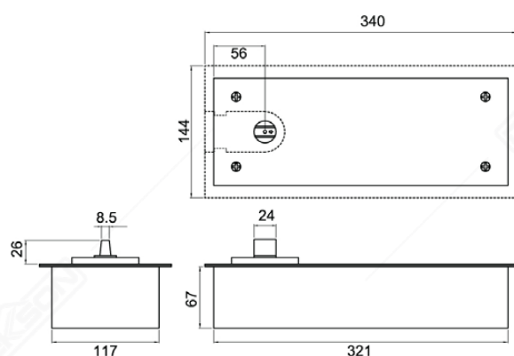
FHA 180 SINGLE SSS Available : FHA 180 DOUBLE SSS
